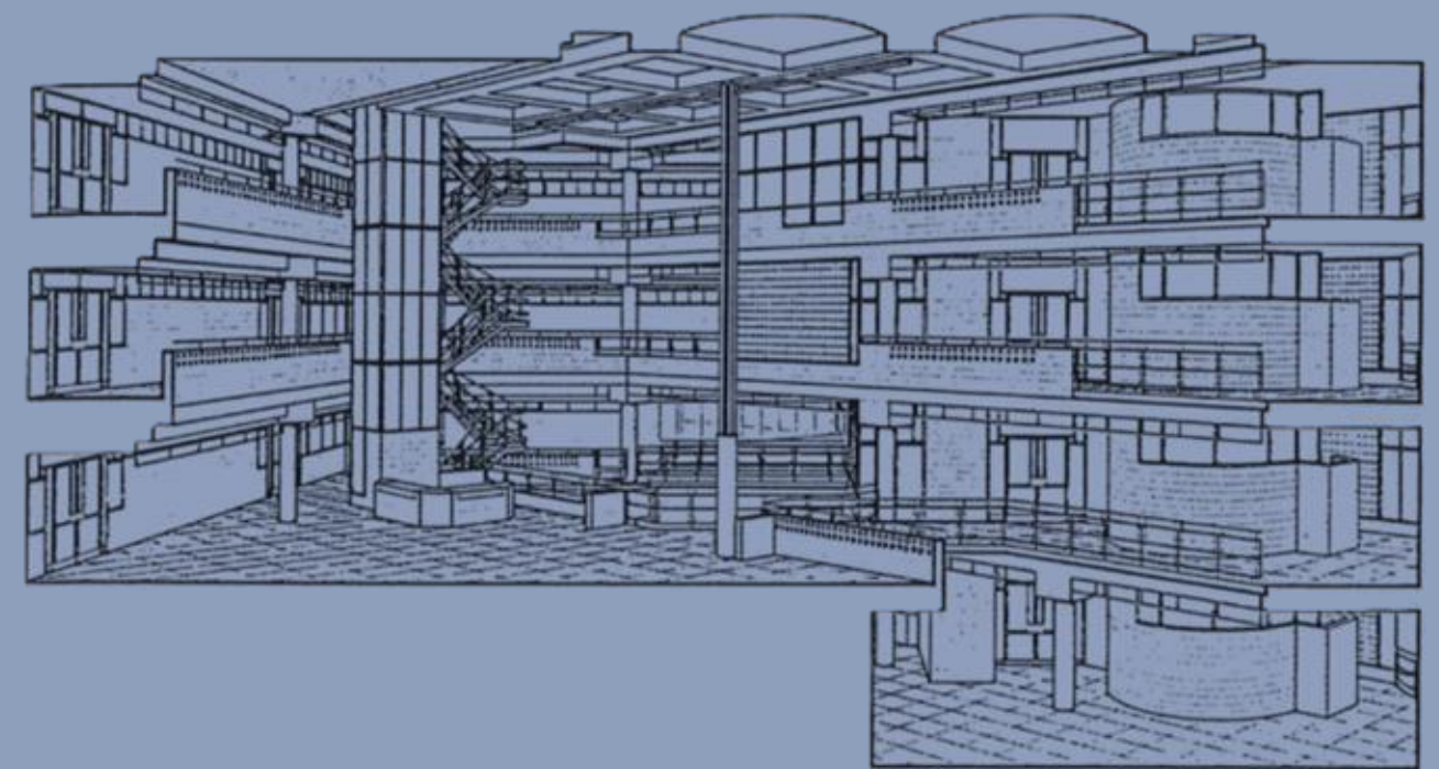
Tettero, W. (Comp.), & Van Duin, L. (Ed.). (1991). Perspectief centrale halruimte [Architectural drawing]. In Ministerie van Sociale Zaken en Werkgelegenheid (Architectonische Studies, 7). Publikatieburo Bouwkunde, Faculteit der Bouwkunde, Technische Universiteit Delft.
